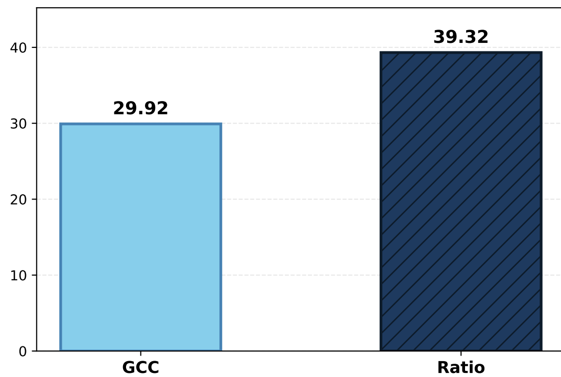
VMAF
