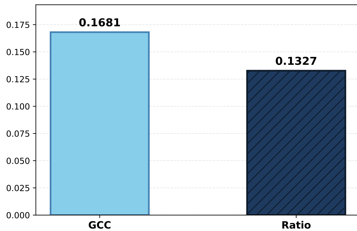
LPIPS
