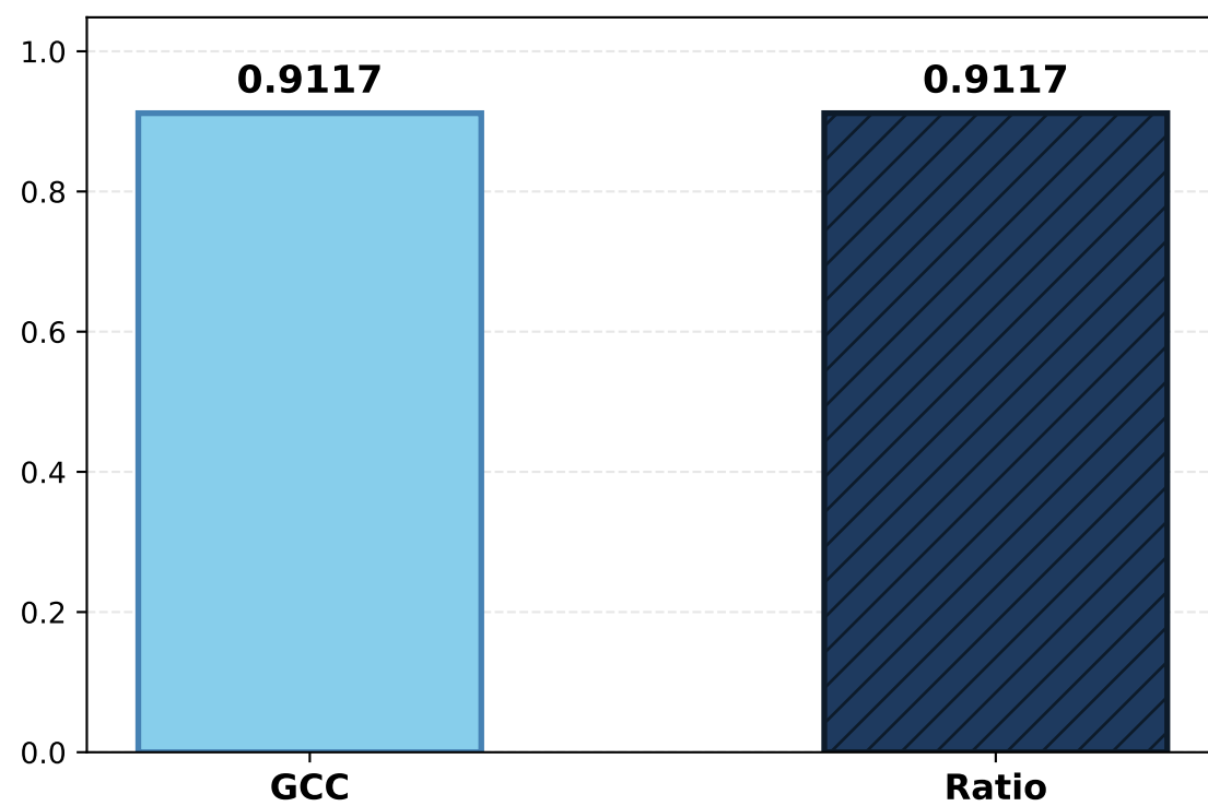
LPIPS
